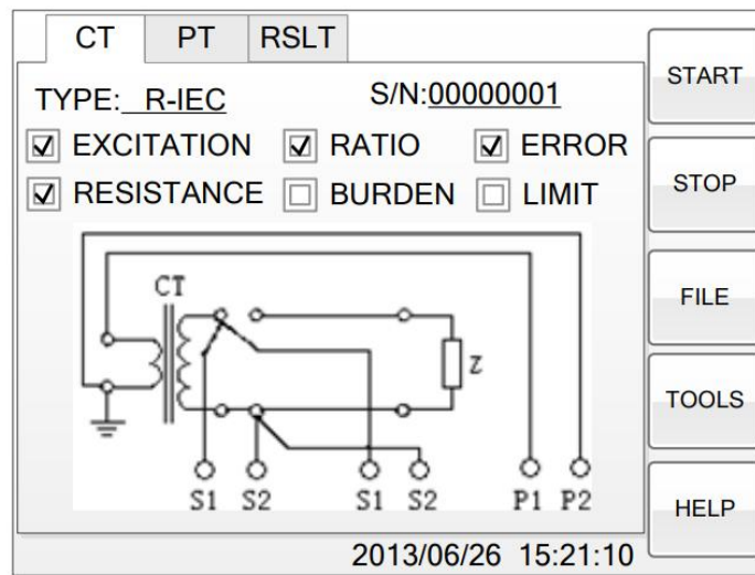
Fig 2.3 Basic parameter Settings interface
